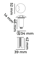
MOL9026 49.00$ SATEN KASA METAL GÖVDE 12 VOLT 1 WATT IP65
