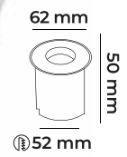
MOL9029 61.00$ SATEN KASA METAL GÖVDE 12 VOLT 1 WATT IP65
